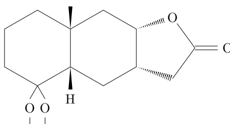
Figure 3 Composé P
