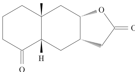
Figure 4 Composé Q
