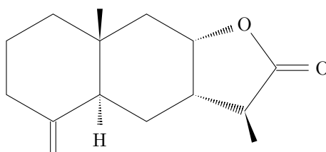
Figure 1 Composé A
