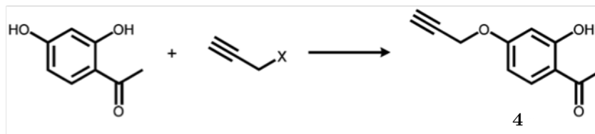
Figure 19 Synthèse de la 2'-hydroxy-4'-propargyloxyacétophénone 4 à partir de paratoluènesulfonate de propargyle \text{HC}\equiv\text{C}-\text{OTs} avec \text{OTs} = \text{OSO}_2 - \text{C}_6\text{H}_4 - \text{CH}_3
