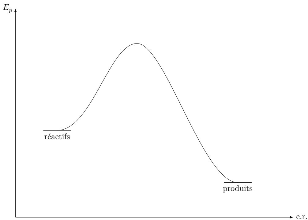
Figure A Profil réactionnel d'une réaction
