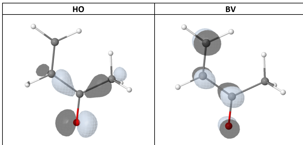
Figure 11 Orbitales frontalières de la buténone
