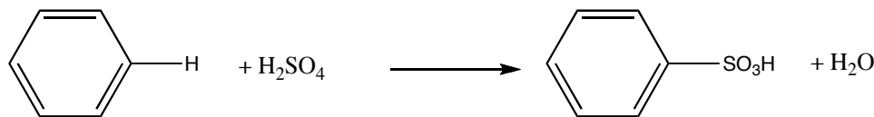
Figure 17 Sulfonation du benzène en acide benzenesulfonique
