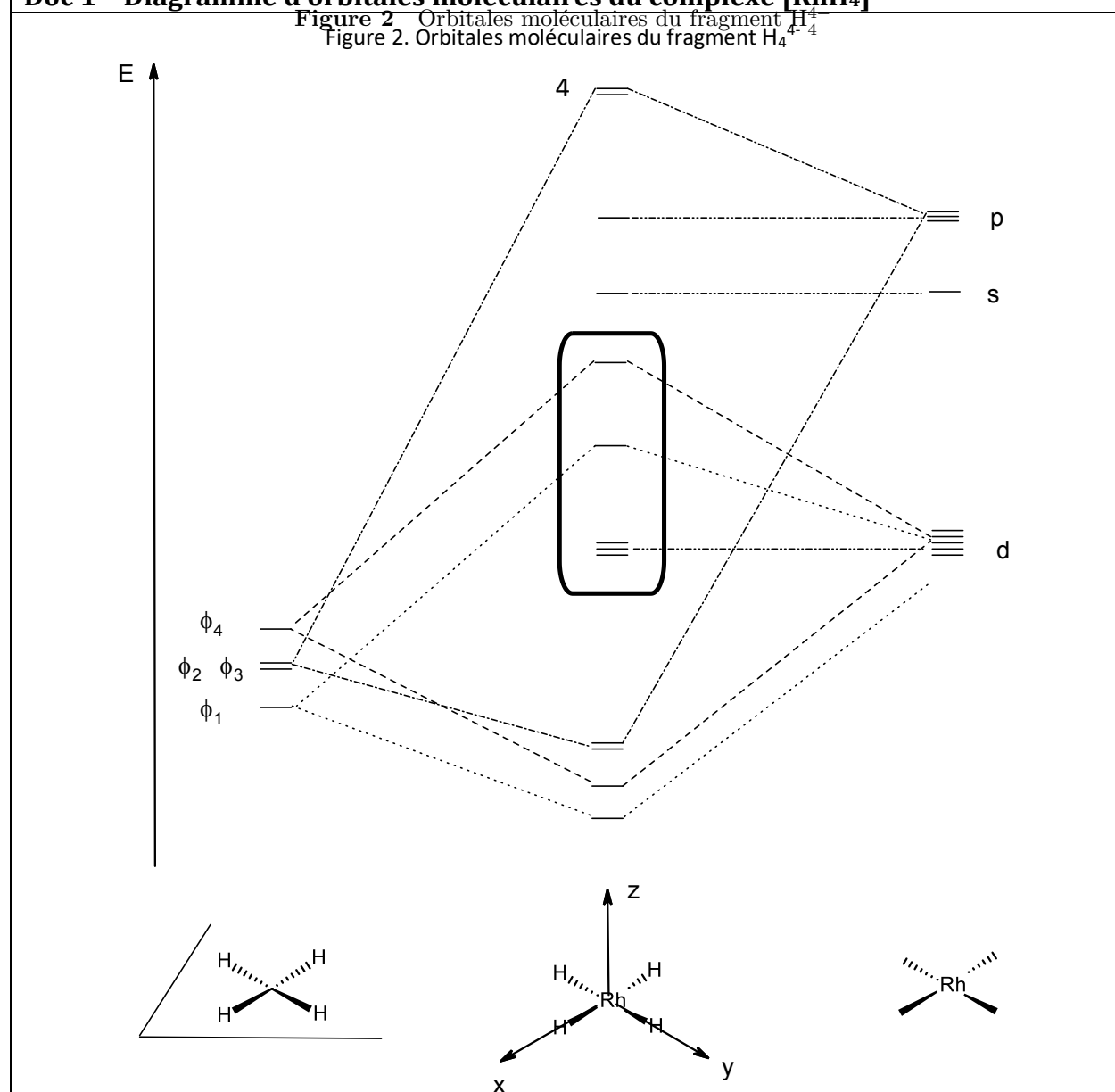
Figure 3 Fragmentation, système d'axes et diagramme d'orbitales moléculaires du complexe [\text{RhH}_4]^{3-} . Les orbitales moléculaires constituant le « bloc d » du complexe sont encadrées.
