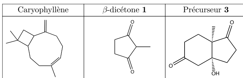
Figure 10 Structures de quelques composés de la synthèse
