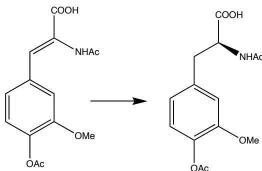
Figure 8 Étape-clé de la synthèse de la L-Dopa
