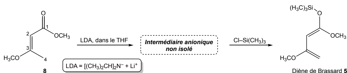
Figure 11 Préparation du diène de Brassard
