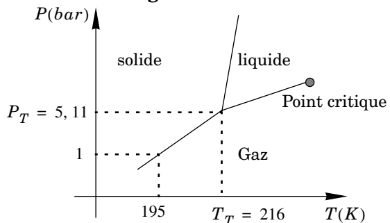
Diagramme de phase du \text{CO}_2 .
