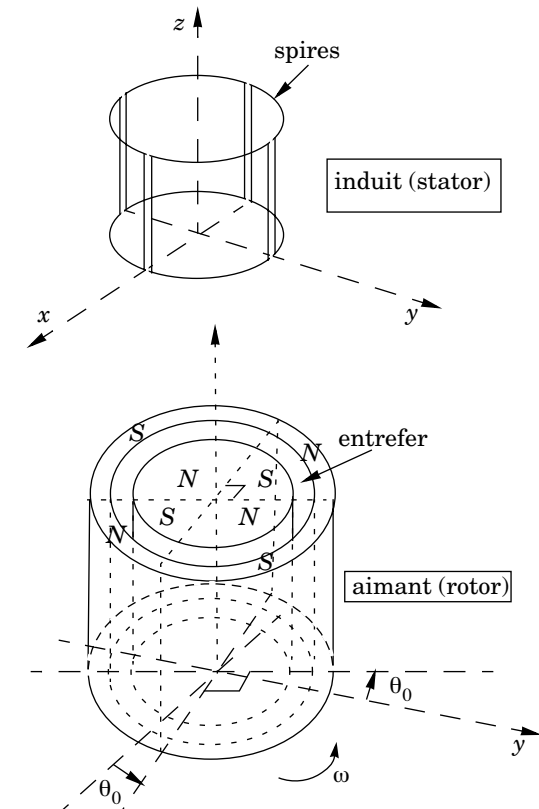
Figure 1 : vue générale Les spires sont représentées hors de l'entrefer
