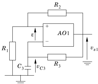
Schéma 5 : comparateur astable
