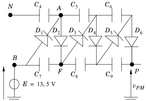
Schéma 7 : multiplicateur de Schenkle
