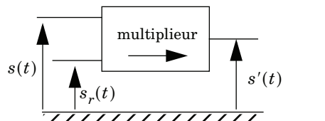
Figure 3 - Principe de la mesure de f_r - f
