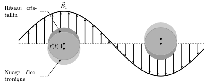
Figure 4 Représentation schématisée des oscillations de plasmon pour une nanoparticule sphérique, montrant le déplacement des électrons libres par rapport au réseau cristallin des noyaux métalliques
