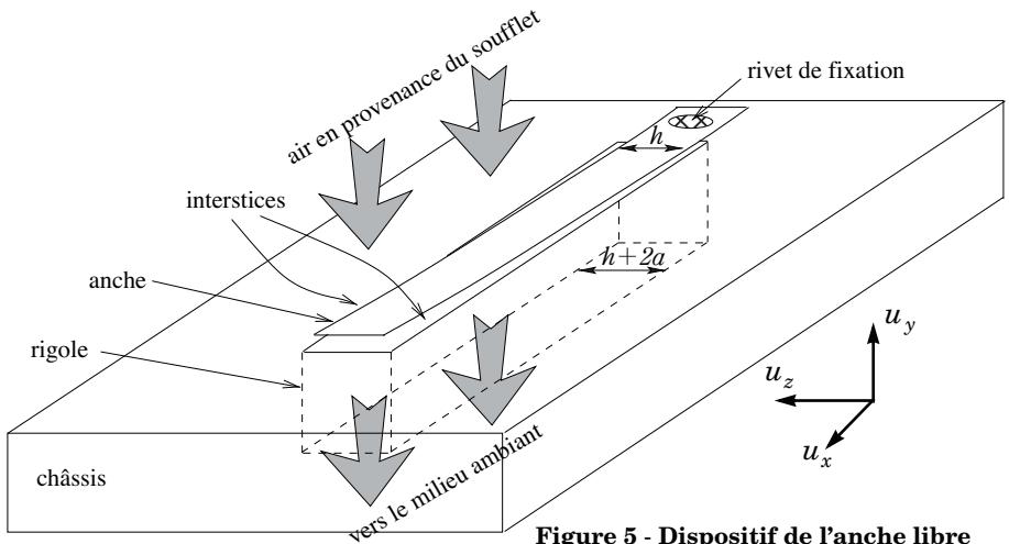
Figure 5 - Dispositif de l'anche libre
