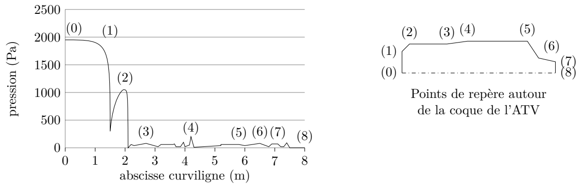
Figure 8 Pression autour de l'ATV à 75 km d'altitude
