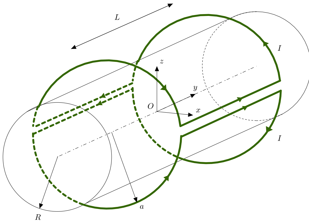
Figure 2 Canalisation entourée d'une bobine de débitmètre électromagnétique
