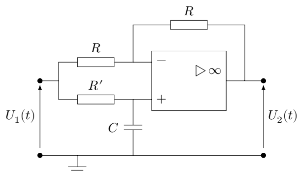
Figure 9 Montage permettant de synthétiser U_2(t)
