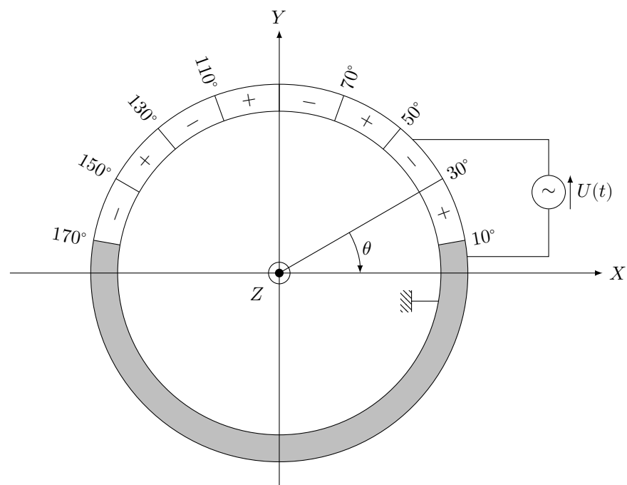
Figure 7 Anneau exciteur constitué d'entités piézoélectriques permettant de générer une onde stationnaire dans l'anneau statorique
