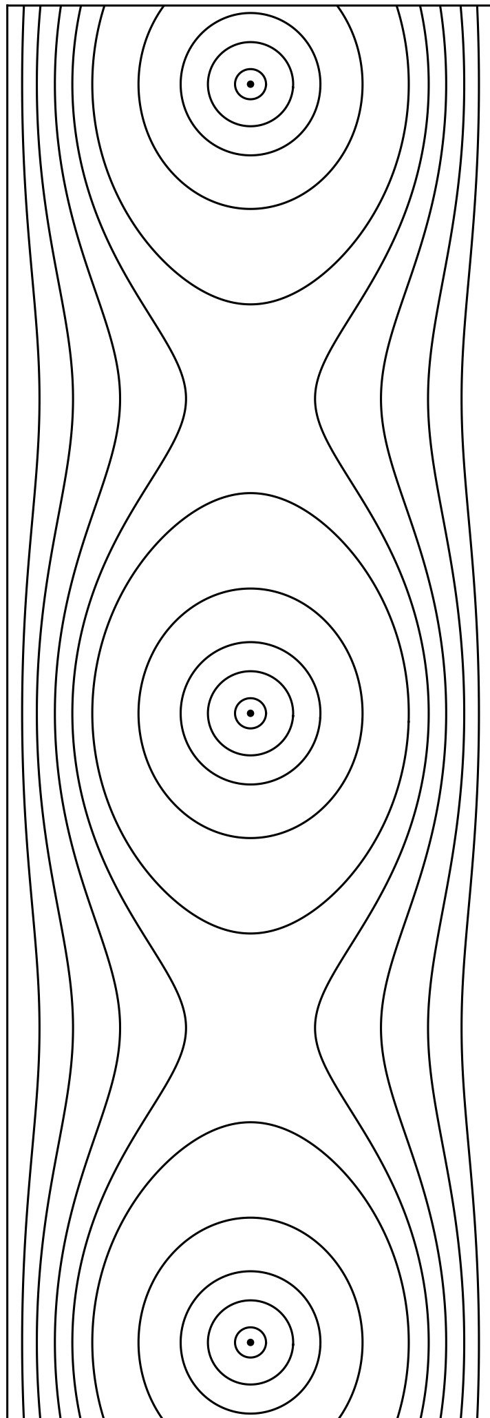
Figure B Carte des équipotentiels dans un électrofiltre sec Téléchargé gratuitement sur www.prepary.fr
