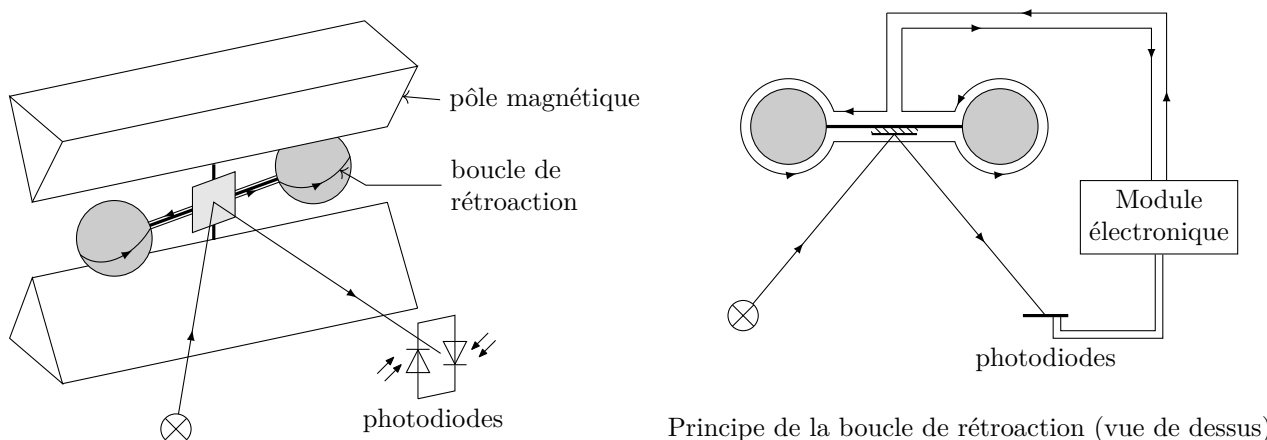
Figure 3 Sonde paramagnétique
