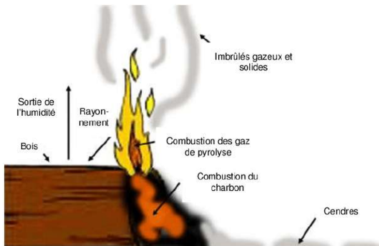
Figure 1 Différentes phases de combustion du bois 1
