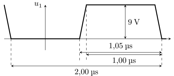
Figure 5 Forme du signal d'entrée u_1
