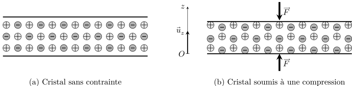
Figure 7 Cristal piézoélectrique
