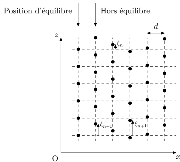
Figure 2 Représentation schématisée des déplacements atomiques.
