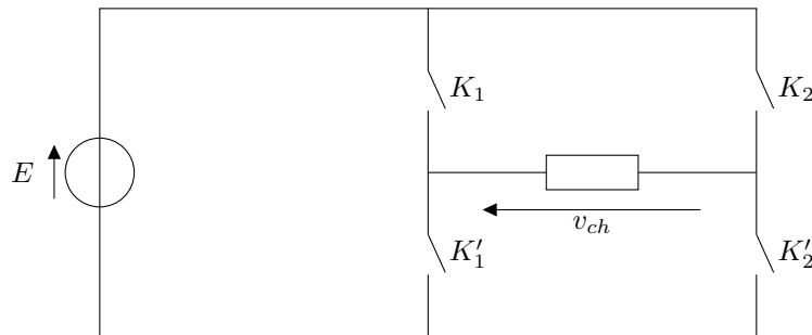
Figure 16 – Onduleur MLI.
