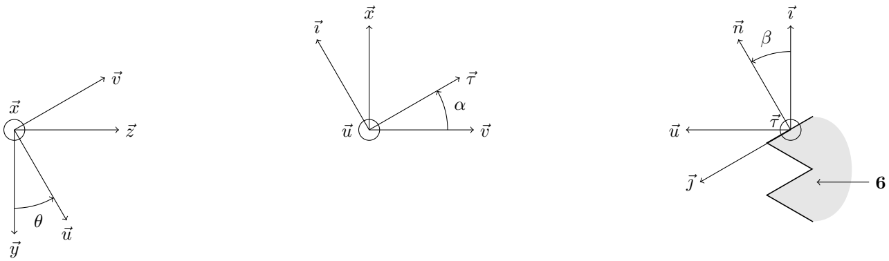
Figure 19 Paramétrage de la liaison hélicoïdale
