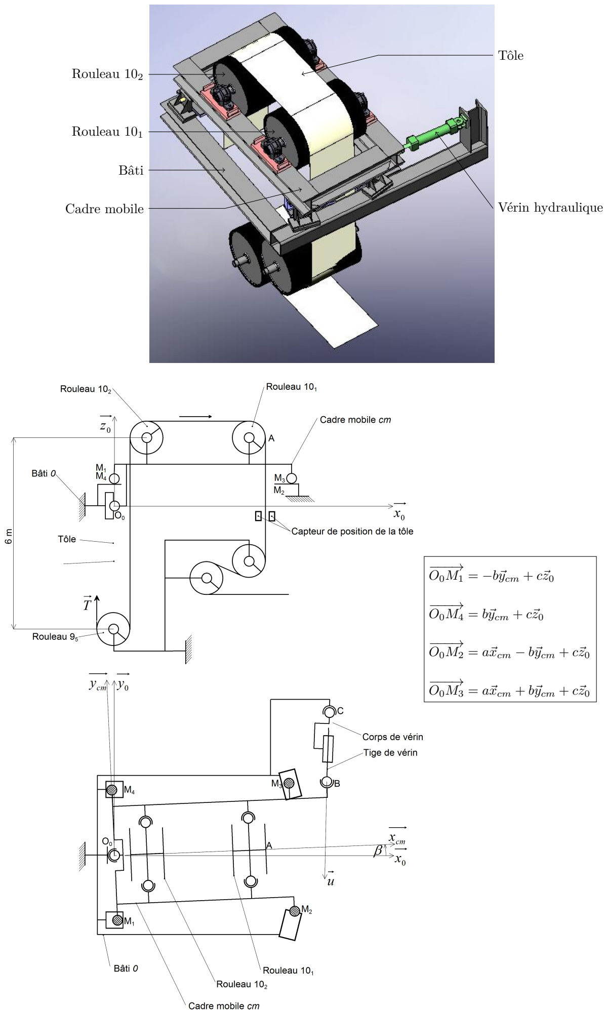
Figure 18 Orienteur d'entrée
