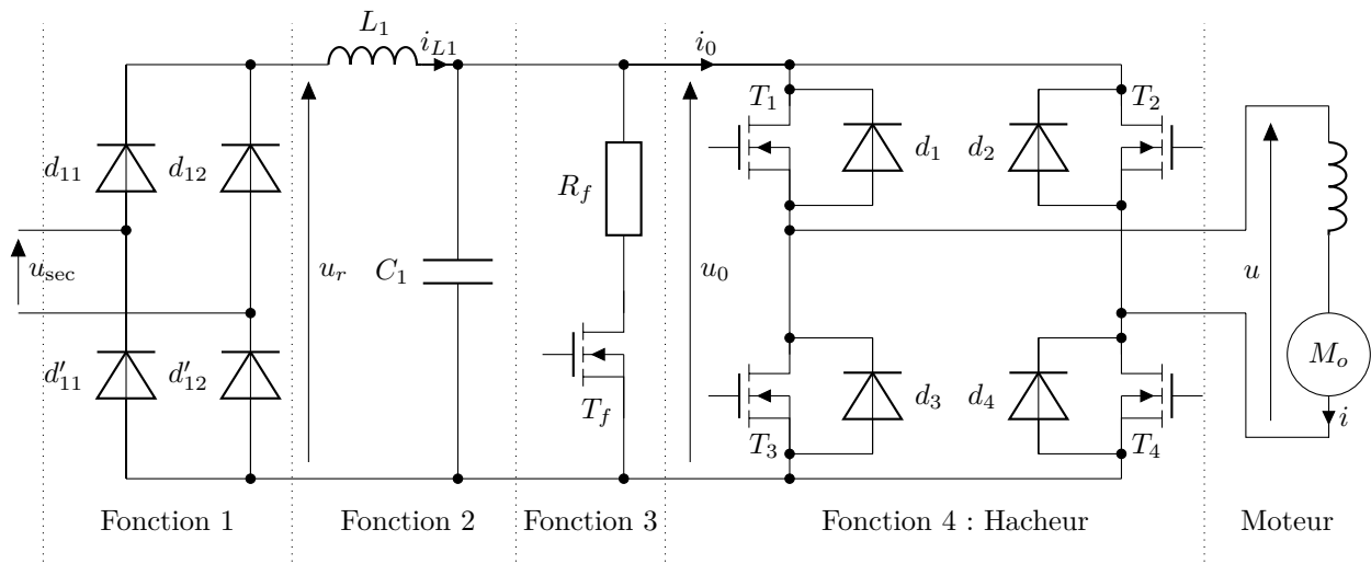
Figure 3 Variateur
