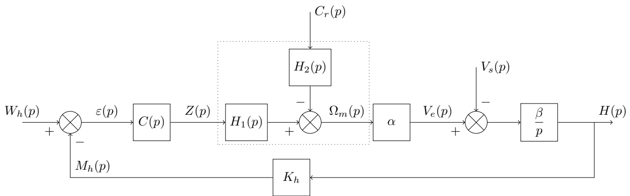
Figure 7 Schéma bloc
