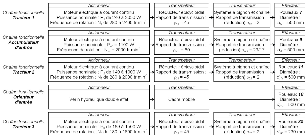
Figure 1 Chaînes d'énergie
