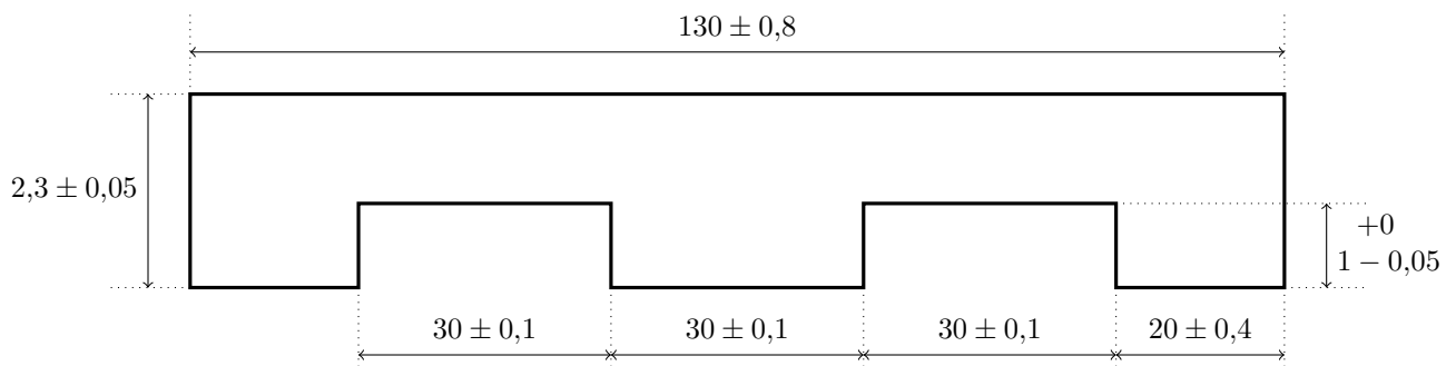
Figure 19 Profil de bande étudié pour le détensionnement
