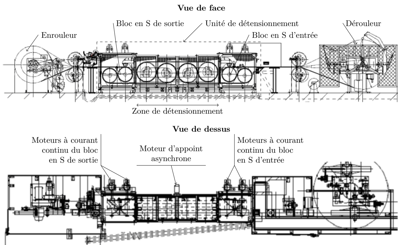
Figure 15 Schéma d'implantation de la ligne de détensionnement
