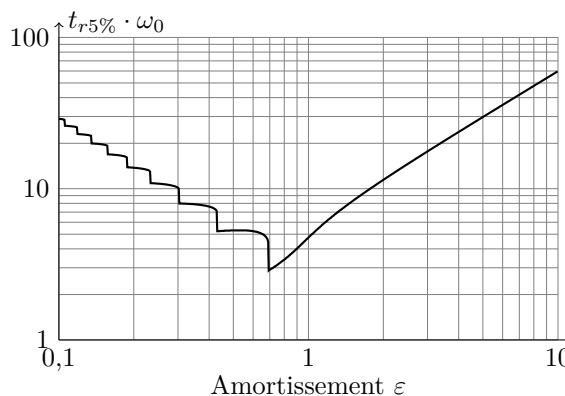
Figure 6 Abaque : produit t_{r5\%} \cdot \omega_0 où t_{r5\%} est le temps de réponse à 5% d'un second ordre de pulsation propre \omega_0 , en fonction de son amortissement \varepsilon
