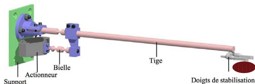
Figure 2 Représentation du stabilisateur actif
