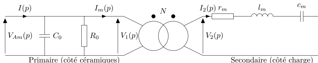
Figure 10 Schéma équivalent de l'actionneur piézoélectrique mécaniquement chargé
