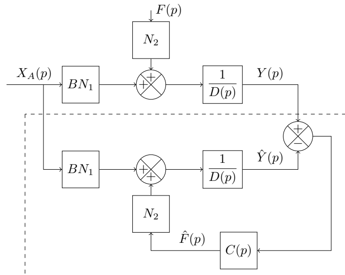
Figure 28 Schéma-bloc du modèle d'estimation de F(p)
