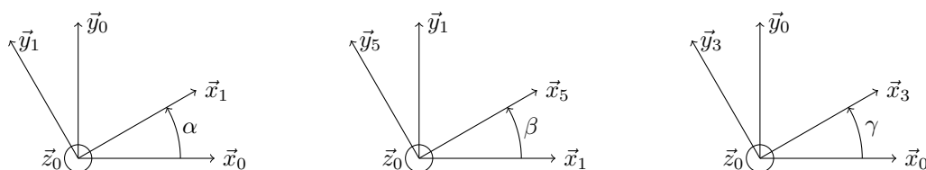
Figure 6 Paramétrage des rotations
