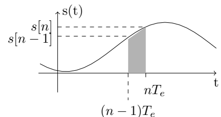
Figure 21 Illustration de la discrétisation par la méthode des trapèzes
