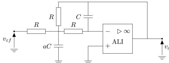
Figure 20 Cellule élémentaire du filtre anti-repliement
