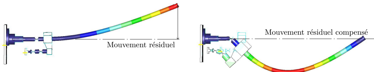
Figure 9 Compensation du mouvement résiduel
