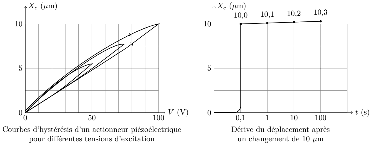
Figure 12 Représentation des phénomènes d'hystérésis et de fluage
