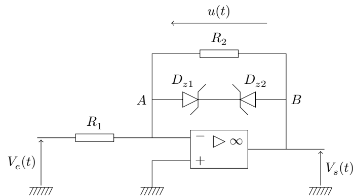
Figure 13 Amplificateur écrêteur
