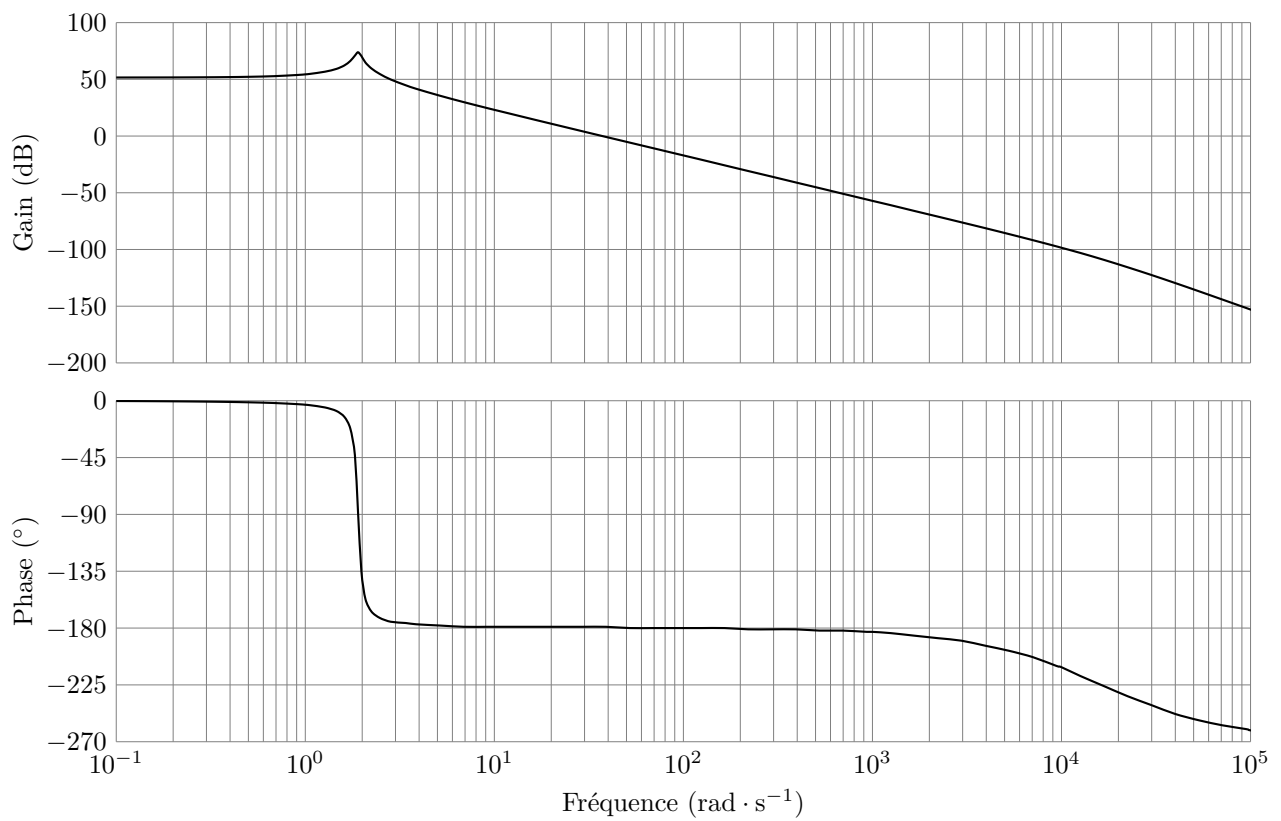
Figure 16 Diagramme de Bode en boucle ouverte de la boucle de position F_{\text{TBO}}(p)
