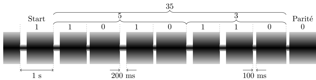
Figure 21 Exemple de trame DCF77 (bits 20 à 28) donnant les minutes (35 ici)
