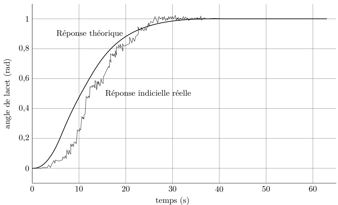
Figure D Réponse indicielle théorique et réelle Télécharge gratuitement sur www.prepary.fr
