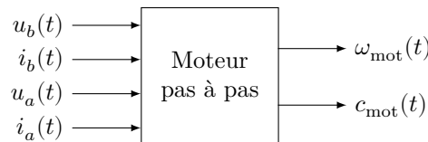
Figure 10 Représentation de l'actionneur dans la base fixe
