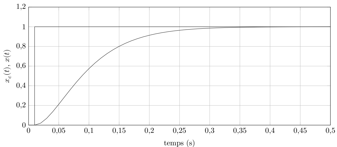
Figure 20 Réponse indicielle de la boucle de position corrigée
