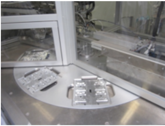
Postes de chargement et de déchargement des plateaux à godets
