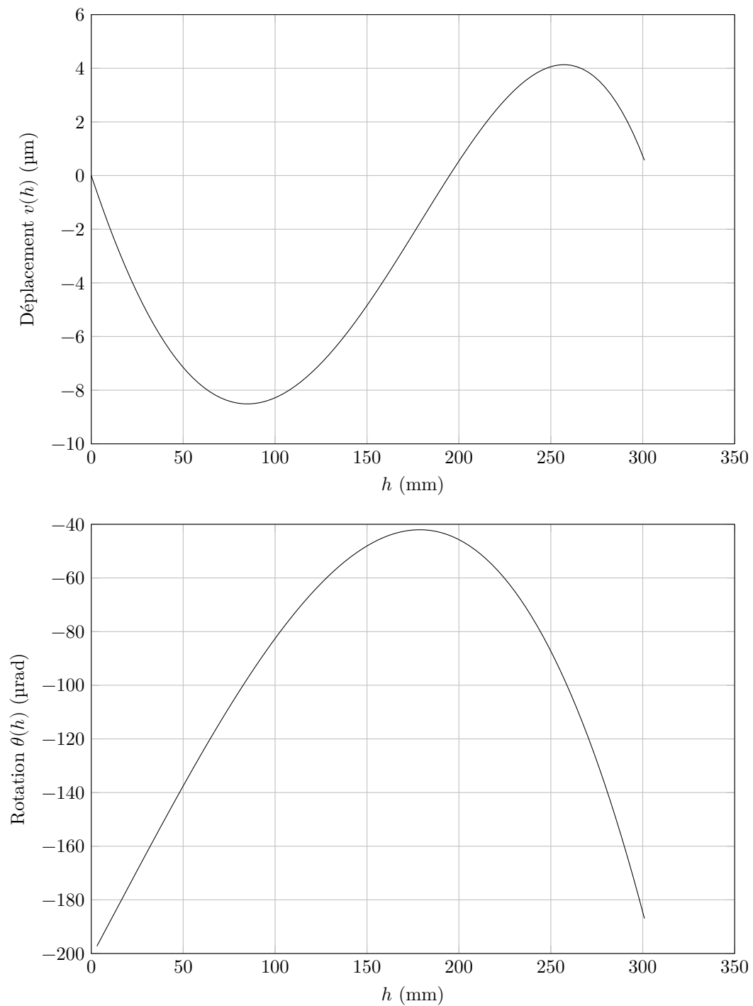
Figure 22 Déplacement et rotation de la section droite de centre H dans le cas où le chariot accélère
