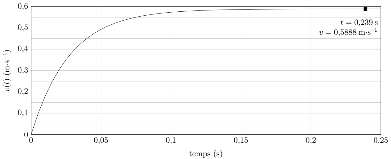
Figure 19 Réponse indicielle de la boucle de vitesse seule non corrigée
