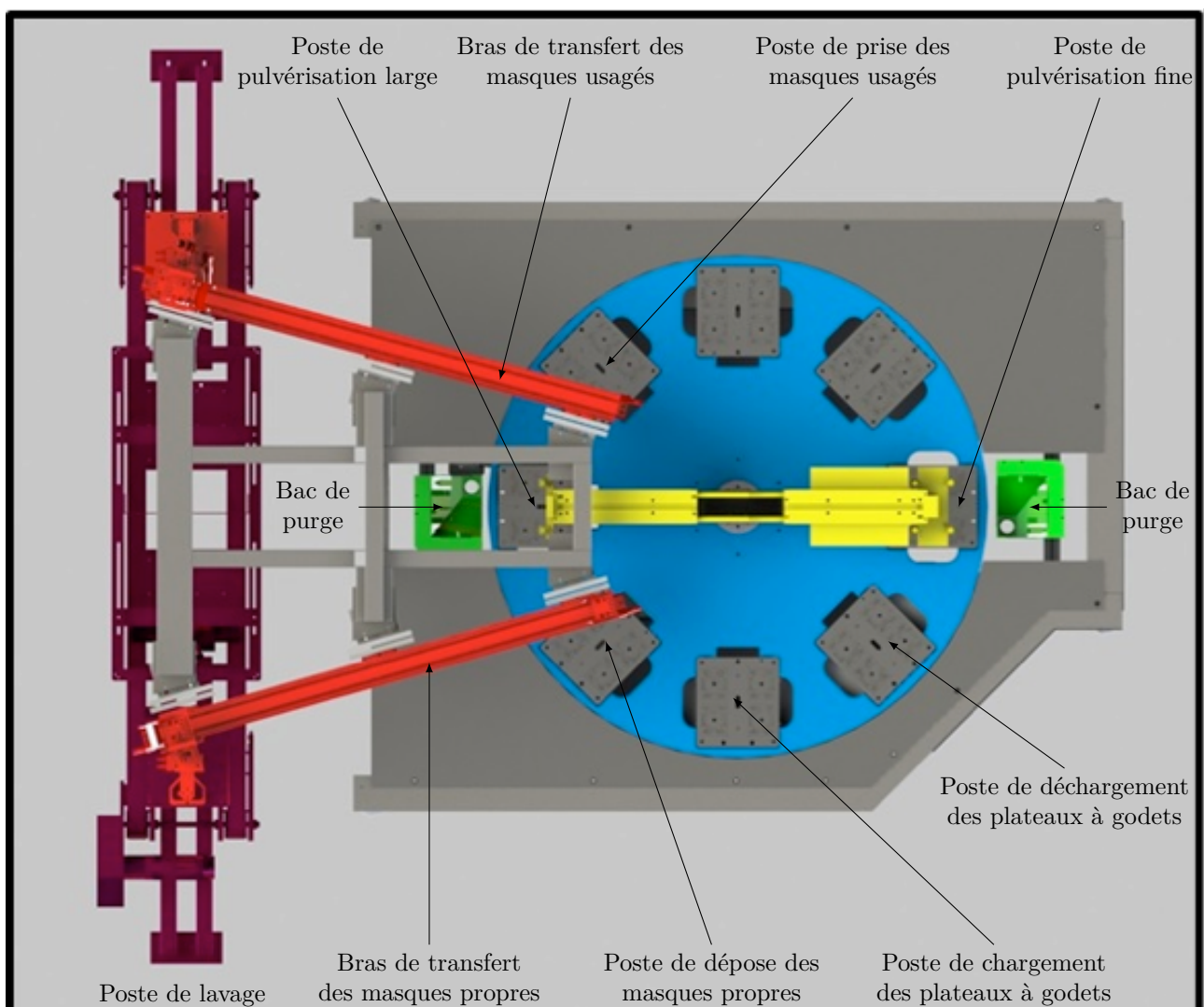
Figure 6 Système de pulvérisation des nacres
