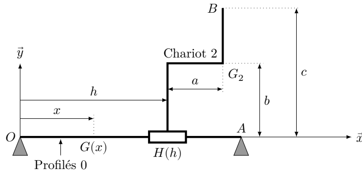
Figure 21 Paramétrage du chariot
