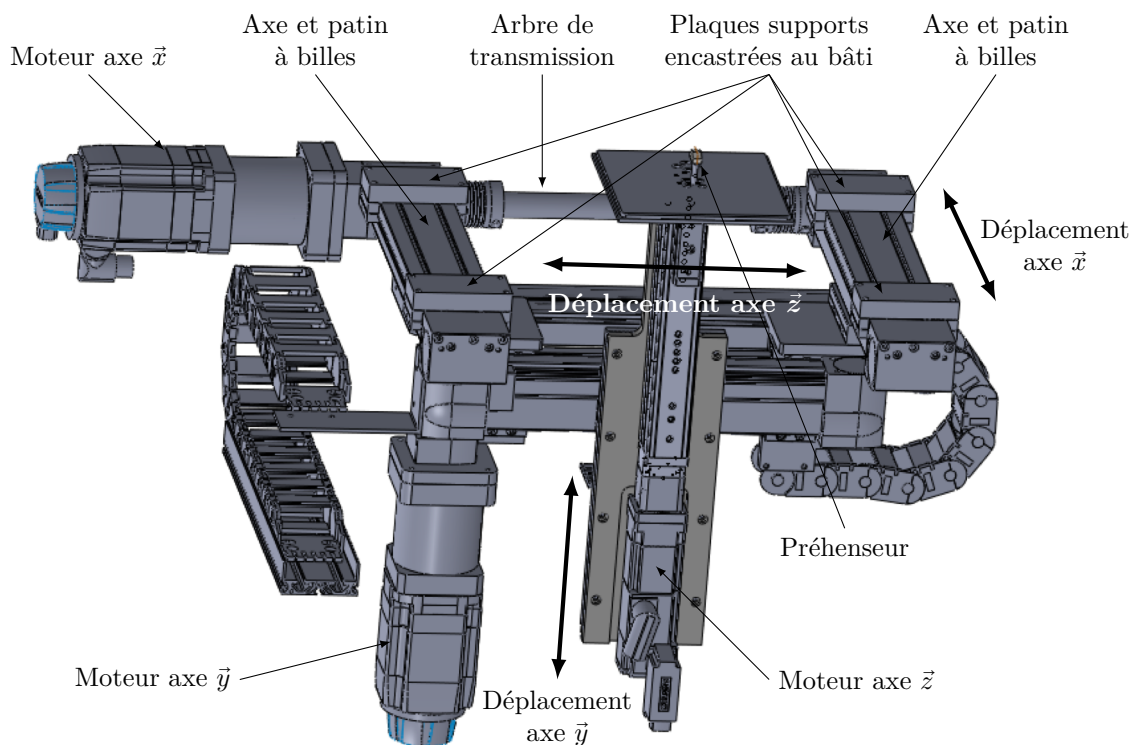
Figure 8 Architecture des différents axes
