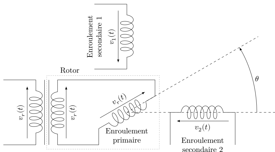
Figure 13 Schéma de principe du résolveur
