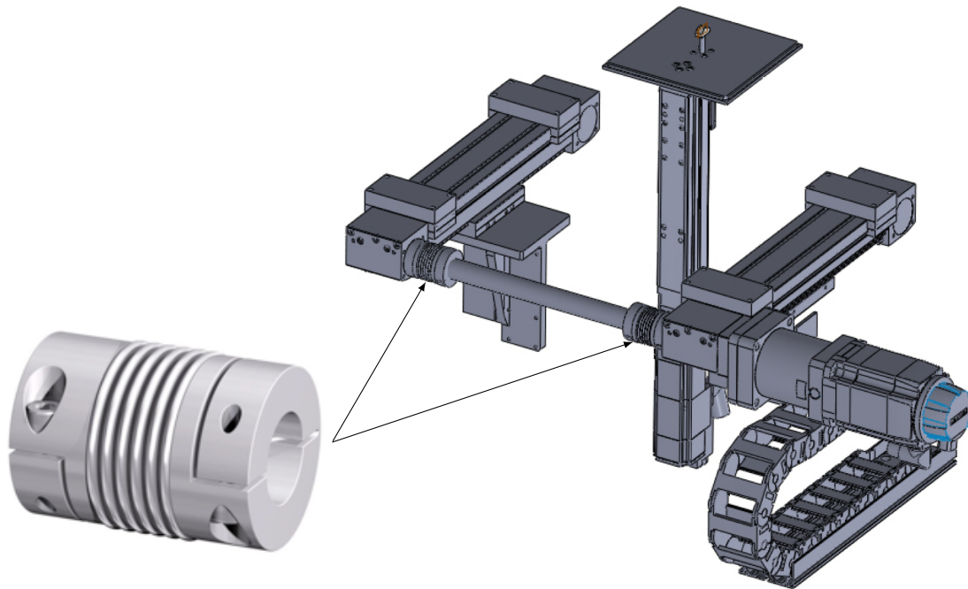
Figure 12 Implantation des soufflets métalliques
