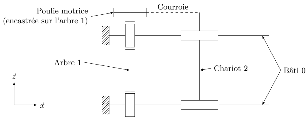
Figure 11 Schéma cinématique de l'axe \vec{x}
