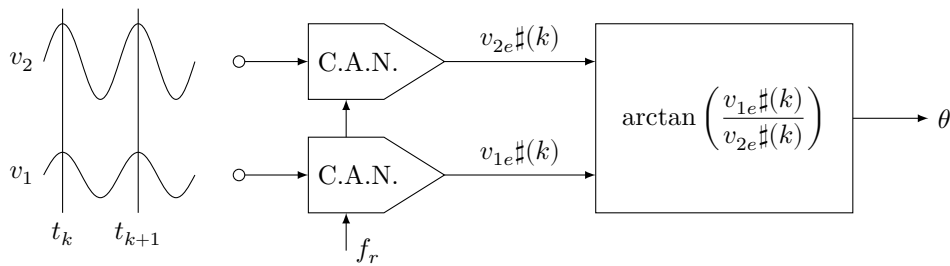
Figure 16 Extraction de la position angulaire du rotor
