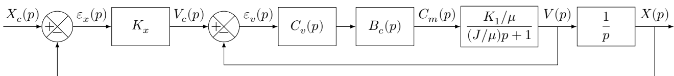
Figure 18 Schéma bloc de l'asservissement de position
