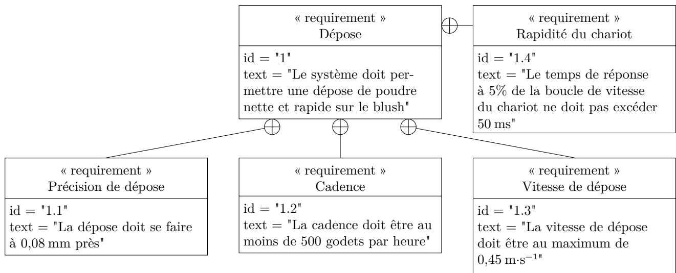
Figure 3 Diagramme des exigences du système
