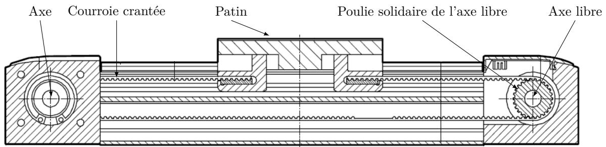
Figure 10 Axe et patin à billes
