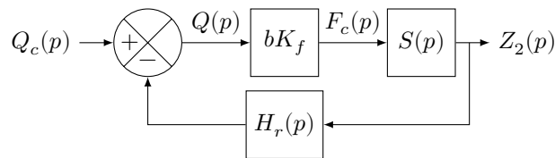
Figure 16 Modèle équivalent de la chaîne d'asservissement complète
