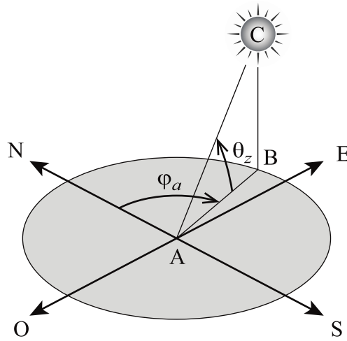
Figure 2 Paramétrage de l'azimut et de l'élévation solaires
