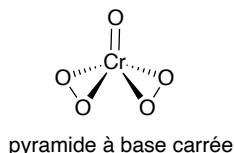
Figure 1. Structure de la molécule \text{CrO}_5 .
