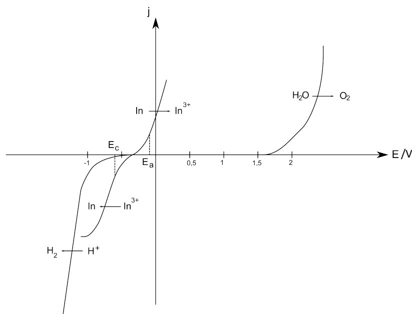
Document 6 : courbes courant-potentiel
