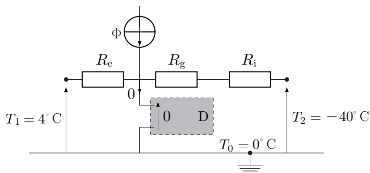
FIGURE 6 – Circuit électrique équivalent à la croissance de la couche de glace. Le dipôle D représenté sur cette figure permet d’assurer une différence de potentiel nulle sans appel de courant dans cette branche du circuit.
