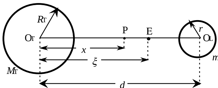
Fig. 1 : notations pour le système Terre-Lune
