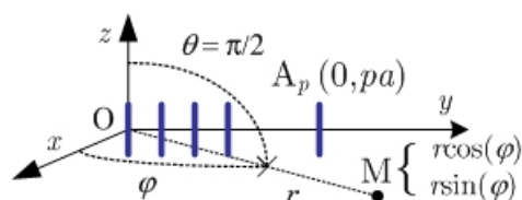
Fig. 12 - Réseau d'antennes demi-onde espacées de « a » sur Oy. Le récepteur est en M (r, phi), dans le plan xOy.
