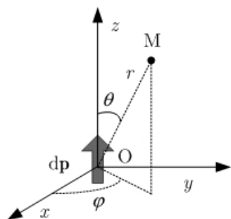
Fig. 7 - Dipole rayonnant.
