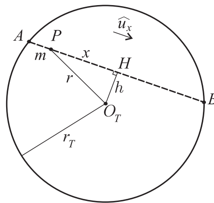
FIG. 1 – Le tunnel droit
