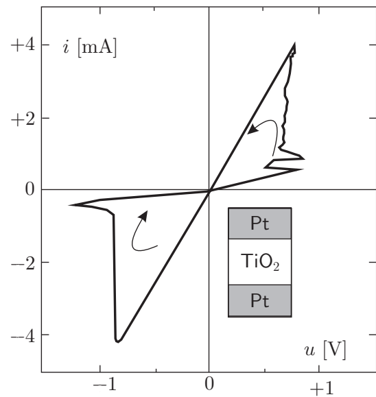
FIGURE 6 – Courbe i(u) expérimentale du film de \text{TiO}_2
