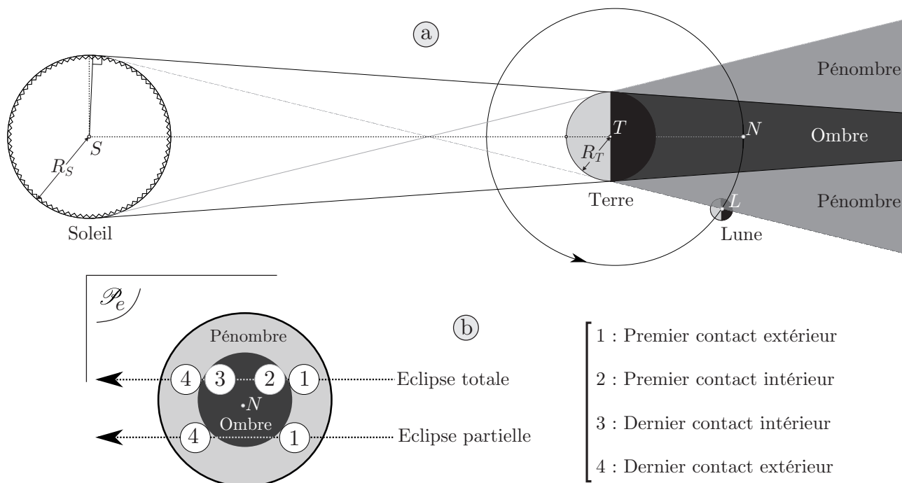
FIGURE 1 – Chronologie d'une éclipse de Lune : a) Phénomène général ; b) Vision depuis la Terre de l'évolution dans une section droite du cône d'ombre terrestre au niveau de l'orbite lunaire. Les disques blancs contenant un chiffre représentent le disque lunaire dans l'étape repérée par ce chiffre
