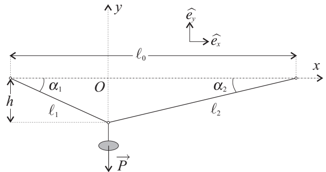
FIGURE 3 – Mesure du module d'Young d'un fil
