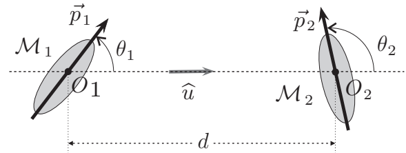
FIGURE 3 – Deux dipôles en interaction
