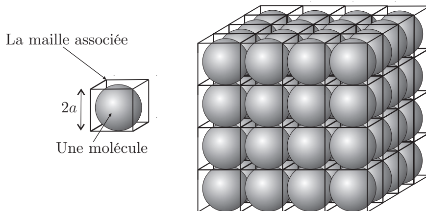
FIGURE 4 – Modèle du liquide pur
