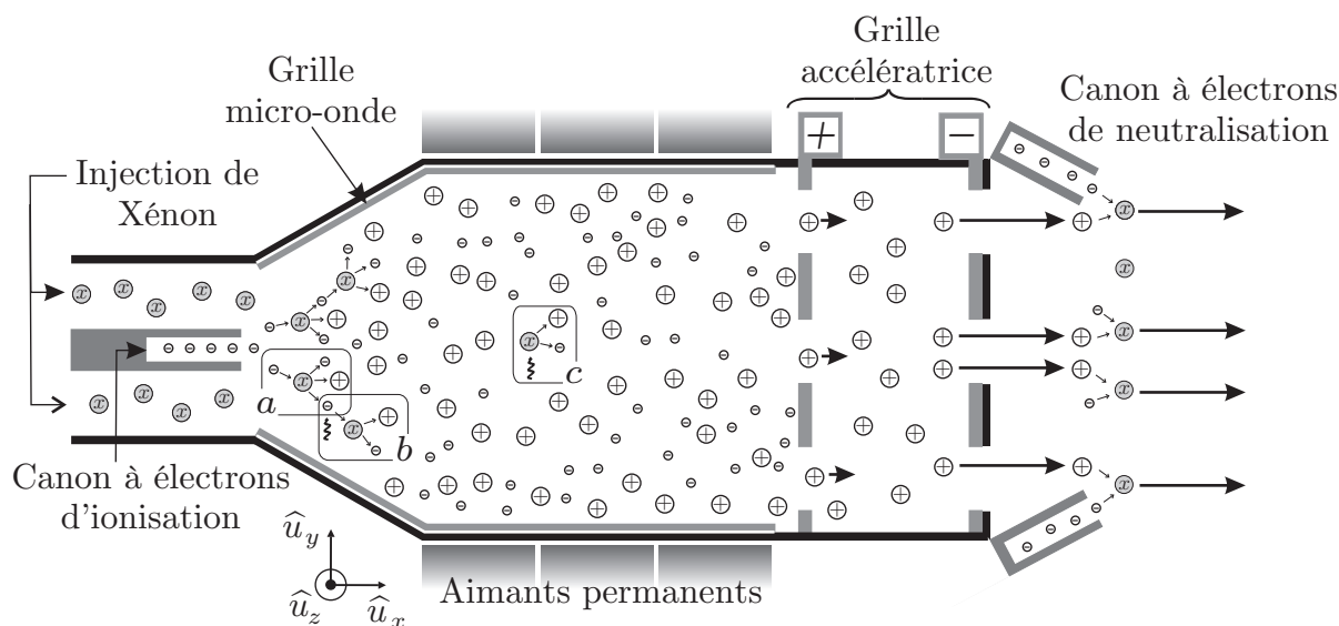
FIGURE 2 — Représentation schématique du moteur ionique : les symboles \otimes sont des atomes de Xénon, \oplus des ions \text{Xe}^+ et \circ des électrons.
