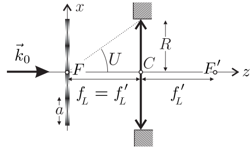
FIGURE 4 – Introduction d'une mire sinusoïdale au foyer.
