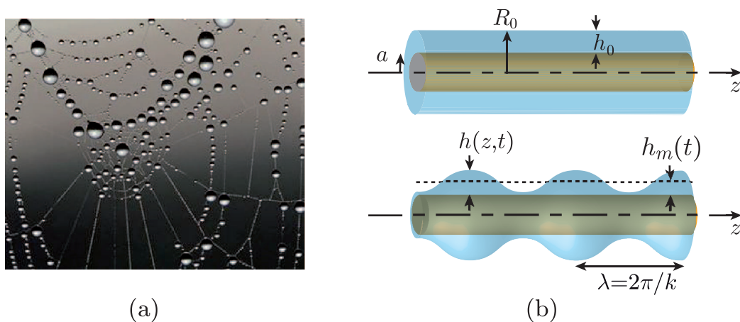
FIGURE 4 – (a) Image tirée de la revue Pour la science , 04 Mars 2010 – (b) Représentation schématique d'une fibre imbibée d'eau.
