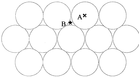
Fig. 4 : Le plan inférieur de l'empilement compact est constitué de sphères dont les centres sont notés A. Une couche identique de sphères, dont les centres sont à l'à-pic des points de type B, est superposée à ce plan. Les centres des sphères de la troisième couche sont en sites de type A, et ainsi de suite (empilement de type ABAB ...).
