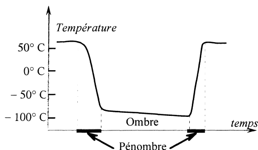
Fig. 3 ; cycle de température lunaire
