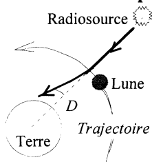
Fig. 5 : Déviation d'un rayon lumineux près de l'occultation
