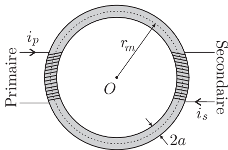
FIGURE 5 — Transformateur
