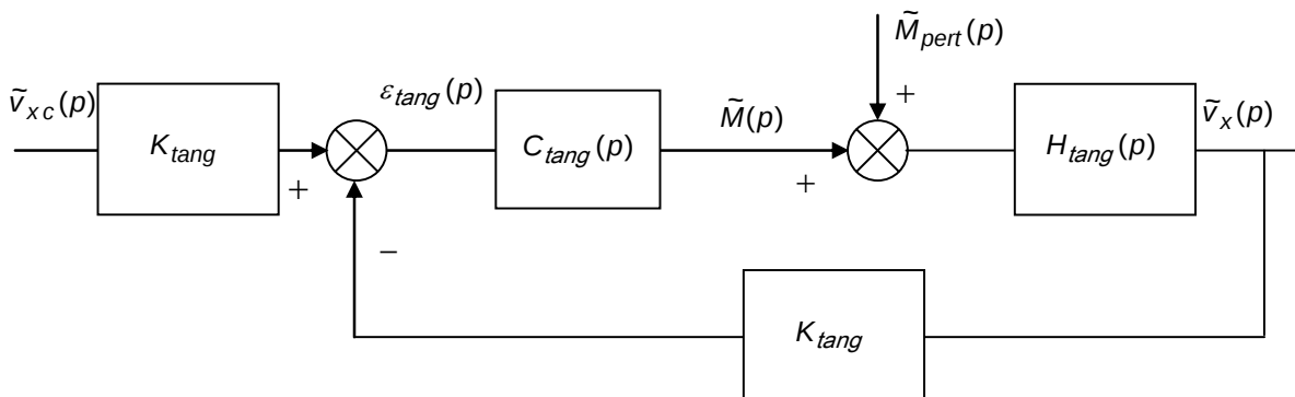
Figure A4 : Schéma-bloc de l'asservissement en tangage
