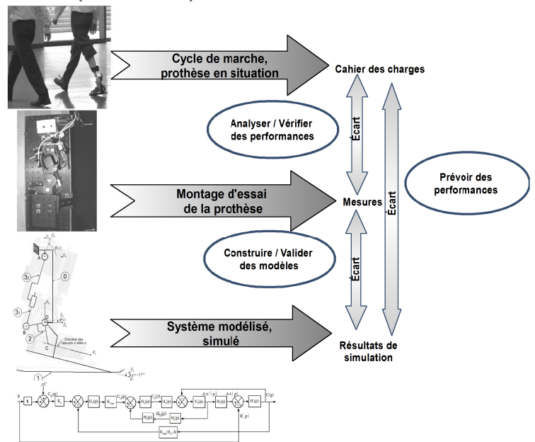
Illustration 4: Démarche d'étude
