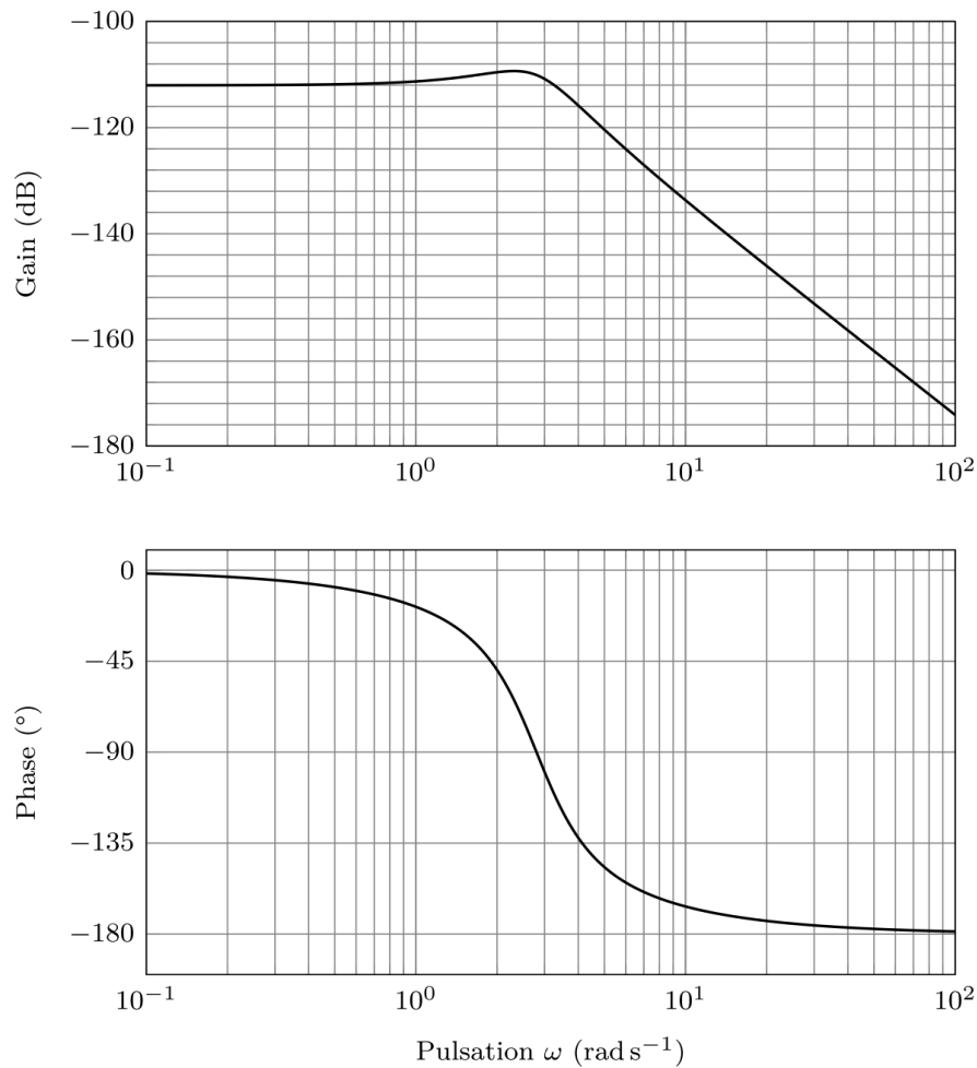
Figure 10 : Diagrammes de Bode de la fonction de transfert H_r(p) . Le module |H_r(j\omega)| est en rad. N -1 . m -1
