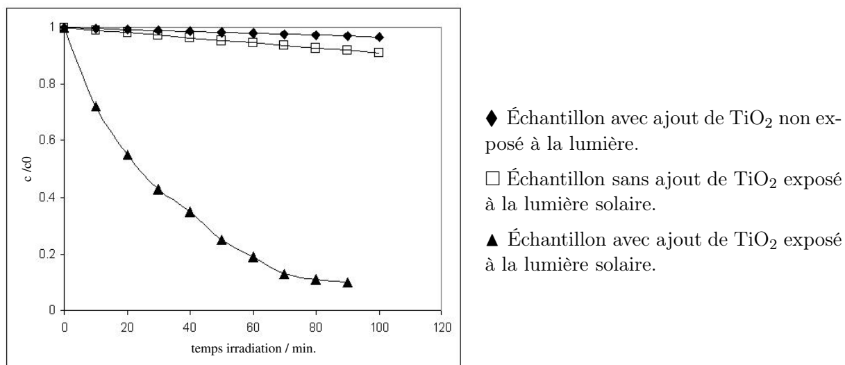
Figure 5 : Évolutions du rapport (C/C_0) en fonction du temps d'irradiation et des conditions (avec C : concentration en AB80 et C_0 : concentration initiale en AB80)
