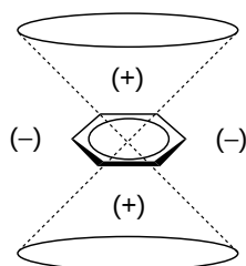
Figure 7 : Partitionnement de l'espace en présence du noyau aromatique
